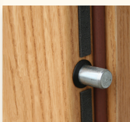
Detail aktivního uzamykacího čepu, protipožární zpěnitelné pásky a obvodového těsnění
