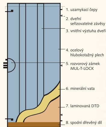
Konstrukce dveří BEDEX STANDARD
